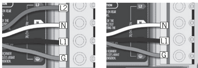
240 V (4 wires)
